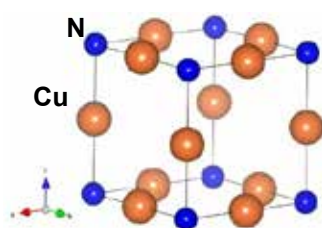
図(a) \text{Cu}_3\text{N} の結晶構造
